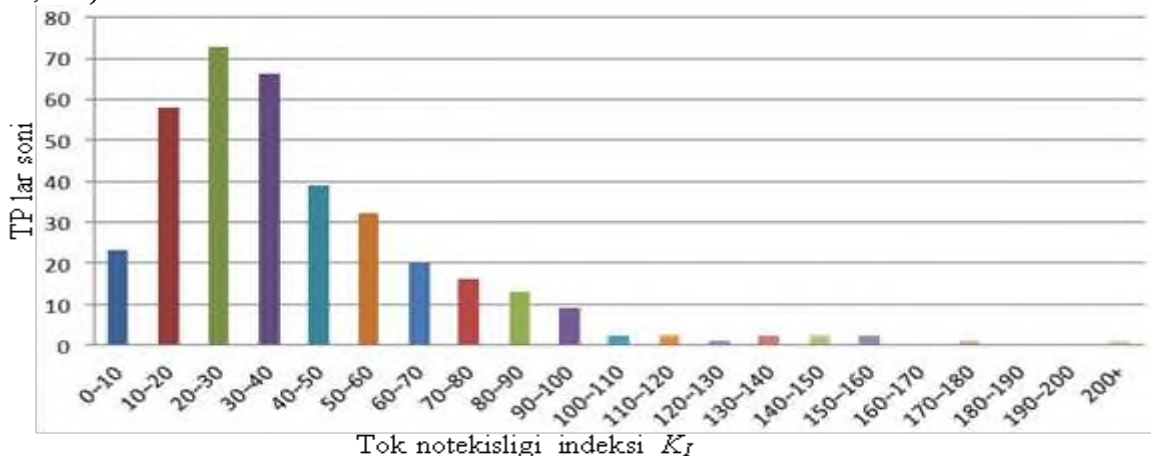
1-rasm. Tok notekisligi indeksi K_I taqsimoti (Navoiy shahar TP lari).
