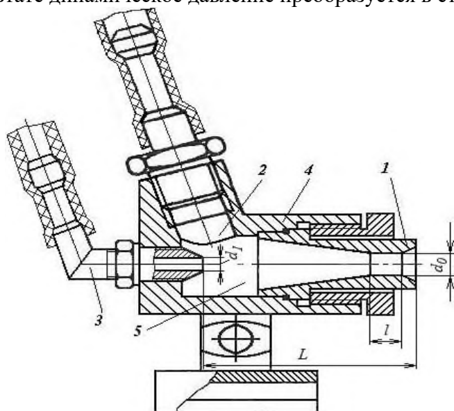
Рис. 1. Конструкция эжектора:
