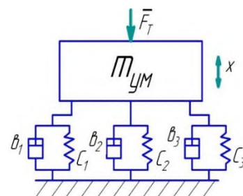
2-rasm. Tavsiya qilingan uch tayanchli, qayishqoq elementli bosh valni vertikal tebranishi hisob sxemasi
