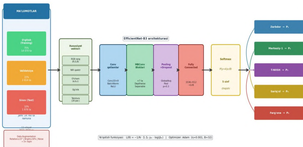
2-rasm. Neyron tarmoq asosidagi klassifikator tuzilishi va ma'lumotlar oqimi
