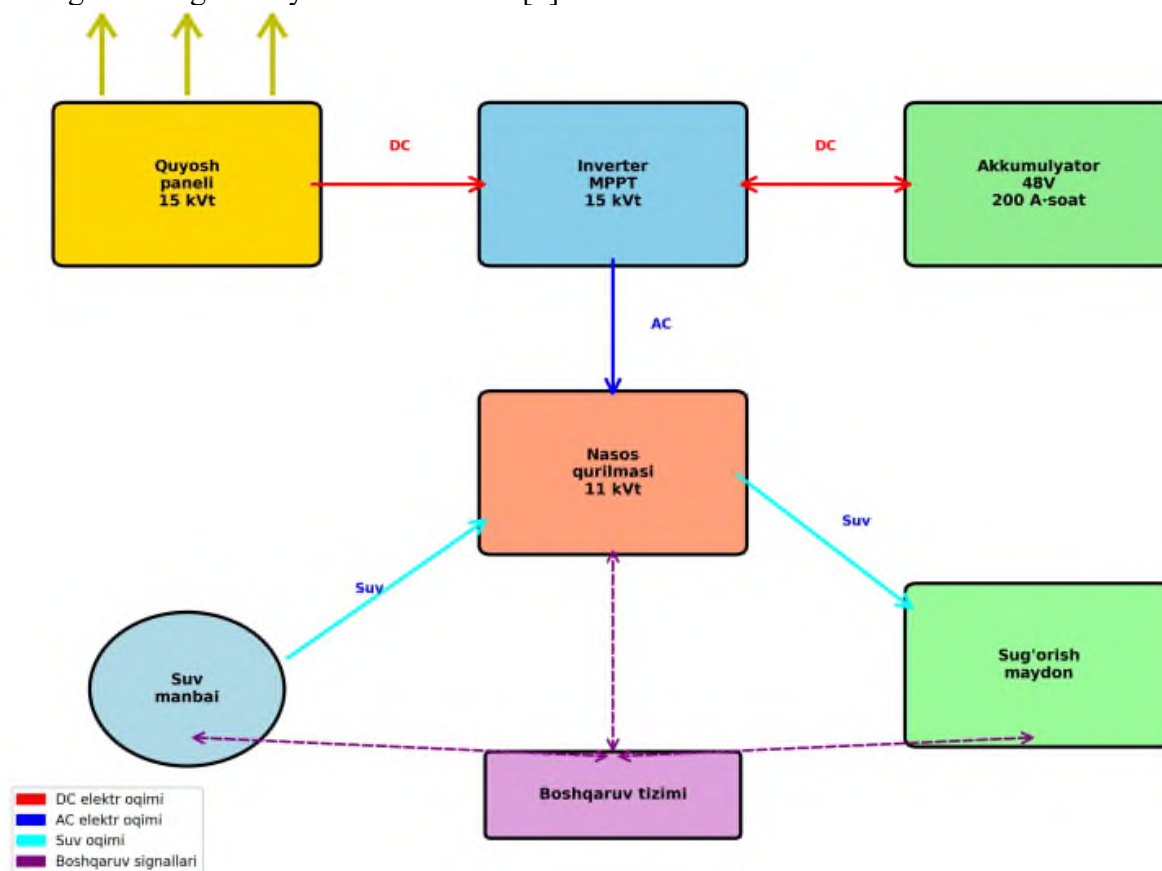
1-rasm. Quyosh panelli nasos tizimining asosiy komponentlari sxemasi
