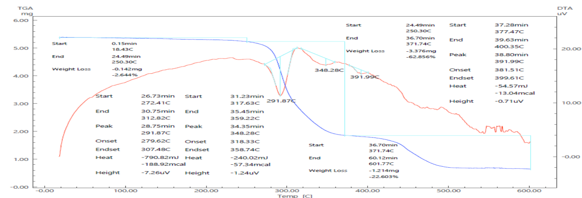
1-рasm. ПBX 1.0 м.б. дериватограммaси. 1- динамик термогравиметрик анализ эгри зиги (ДТГА); 2- динамик термогравиметрик анализ эгри чизигининг ҳосилaси (ДТГП); 3- DSK эгри чизиги.
