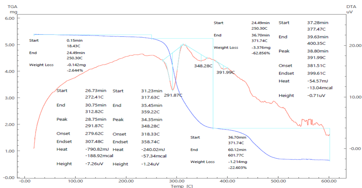
2-расм. ПВХ 2.0 м.б. дериватограммаси. 1- динамик термогравиметрик анализ эгри чизиги (ДТГА); 2- динамик термогравиметрик анализ эгри чизигининг ҳосиласи (ДТГП); 3- DSK эгри чизиги.
