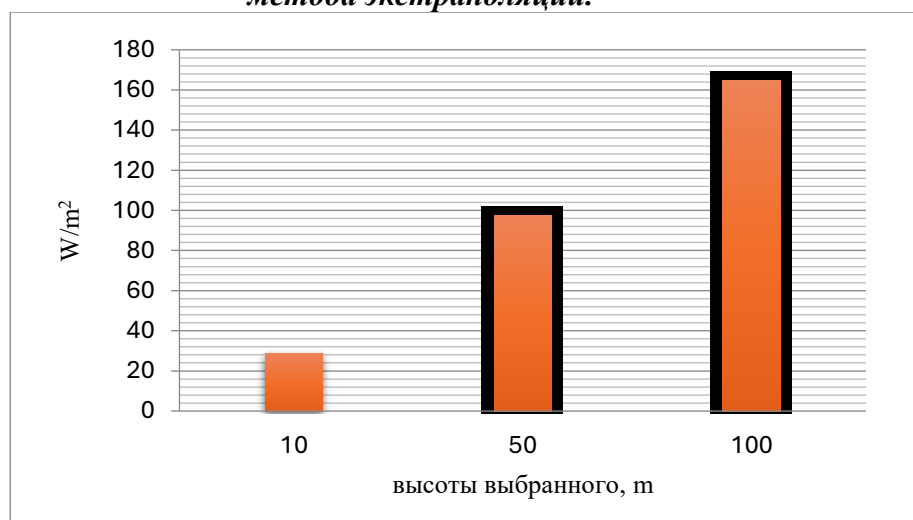
Рис.7. Среднегодовое значение для измеренных по распределению Вейбулла удельной мощности ветра на выбранных высотах.
