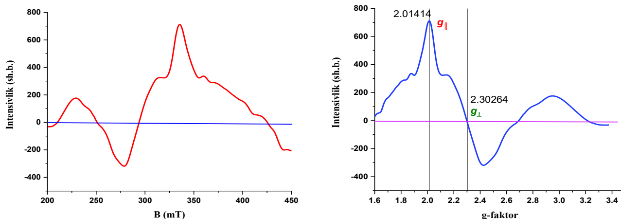
3-rasm. [Co(tmphen)_3](PF_6)_2 kompleksning EPR spektri
