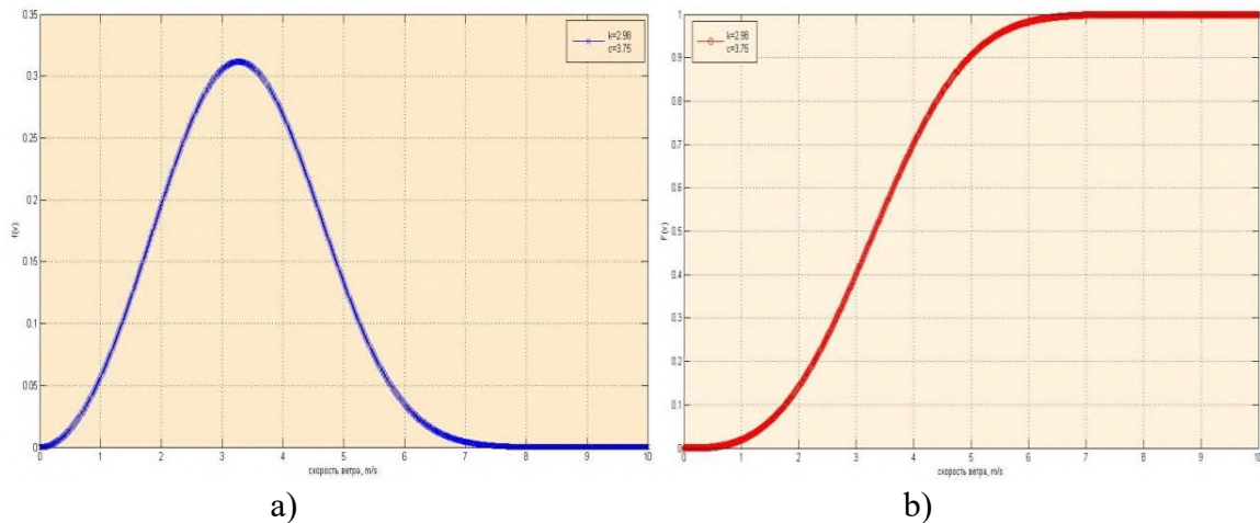
Рис.3. Функция распределения Вейбулла и измеренная плотность (а), интегральная функция распределения Вейбулла со скоростью ветра для выбранных мест на станциях: высота годового показателя и масштабные коэффициенты (б).
