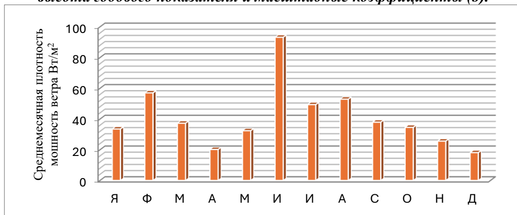
Рис.4. Среднемесячное значение удельной мощности измеренных на основании функции распределения Вейбулла.
