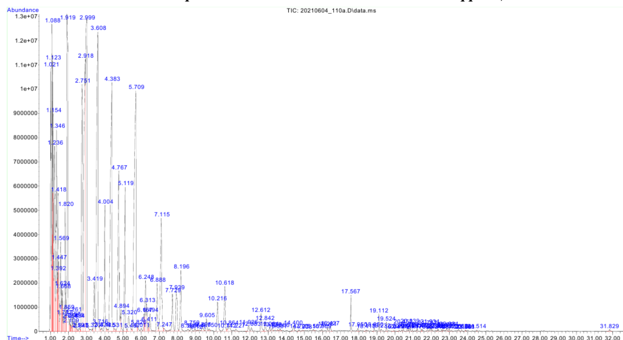
8 – расм. АИ-80 бензинининг 110°С – с.қ.х. фракцияси
