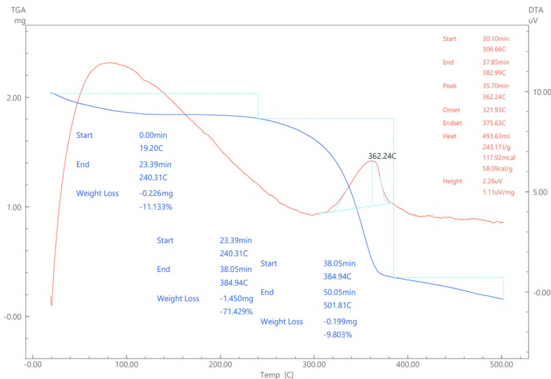
2-rasm. Kislotali usulda olingan sellyuloza TGA va DTA/DSC grafigi
