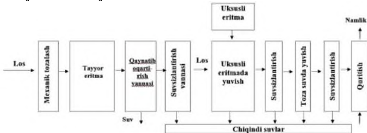
1-rasm. Pilla sannohini qaynatib oqartirish texnologik sxemasi.
