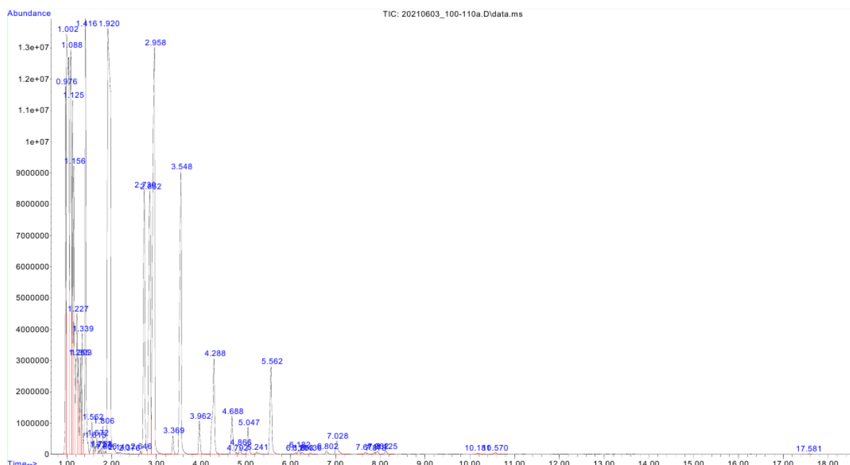
7 – расм. АИ-80 бензинининг 100 – 110°С фракцияси
