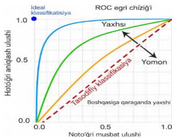
3-rasm. ROC egri chizigʻi
