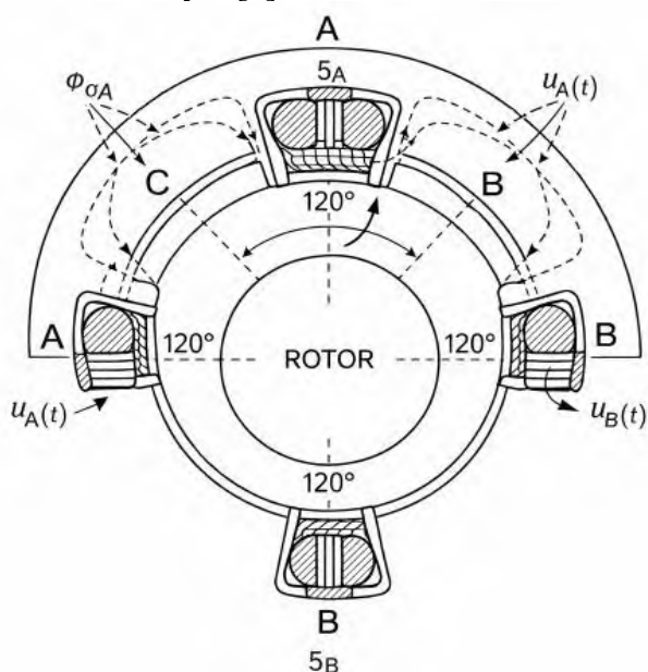
2-rasm. Asinxron motor statorida o'lchov chulg'amlarining uch fazali ( 120^\circ ) joylashuvi va induksiyalangan kuchlanishlar sxemasi
