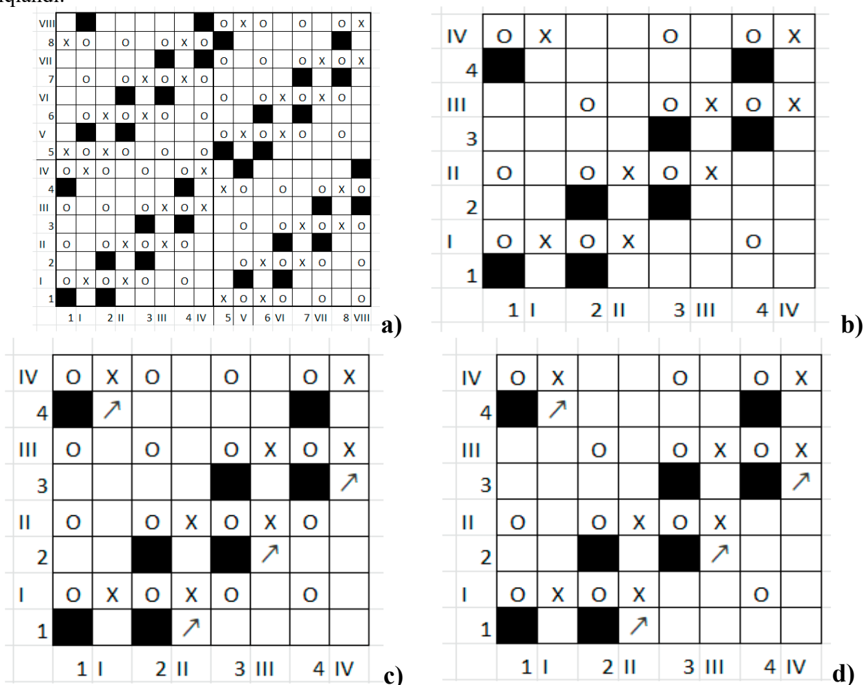
1-rasm. Qatlamlarni birlashtirishning turli usullari bilan ikki qatlamli to'qimaning model o'rilishlari: a) (1-namuna) naqsh konturi bo'yicha, b) (2-namuna), “yuqoridan-pastga” c) (3-namuna) “pastdan-yuqoriga”, d) (4-namuna) kombinatsiyalashgan
