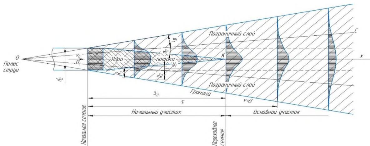
Рис. 2. Схема свободной струи
