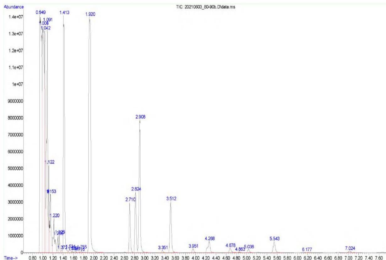
5 – расм. АИ-80 бензинининг 80 – 90°С фракцияси
